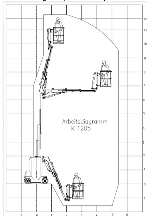
2.2. Arbeitsdiagramm (Arbeitsbereich)
